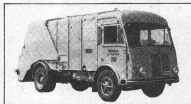
4) FBW L 35 U: Kehrriemwagen Motor: FBW CU (130 PS) Getriebe: Allison MT-41 (Automat)
