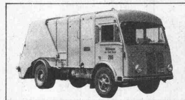
4) FBW L 35 U: Kehrichtwagen Motor: FBW CU (130 PS) Getriebe: Allison MT-41 (Automat)
