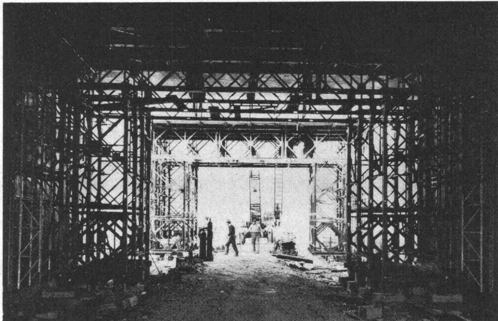
Fahrschalung SBB-Tunnel Gellert-Dreieck Basel Preiswerk + Cle AG Basel
