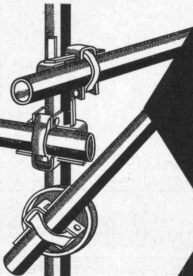
Stahlrohrgerüste KAPPELER
