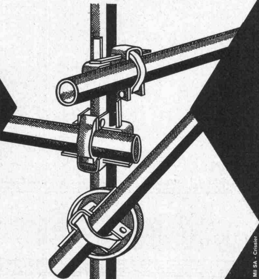
Stahlrohrgerüste KAPPELER
