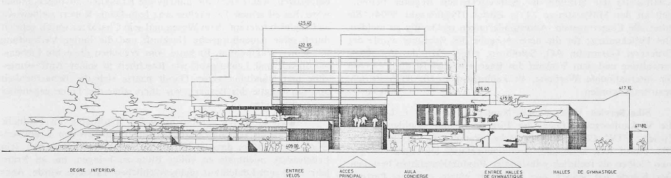
Südvansicht 1:500
