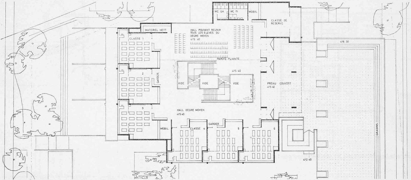
Oberes Eingangsgeschoss 1:500
