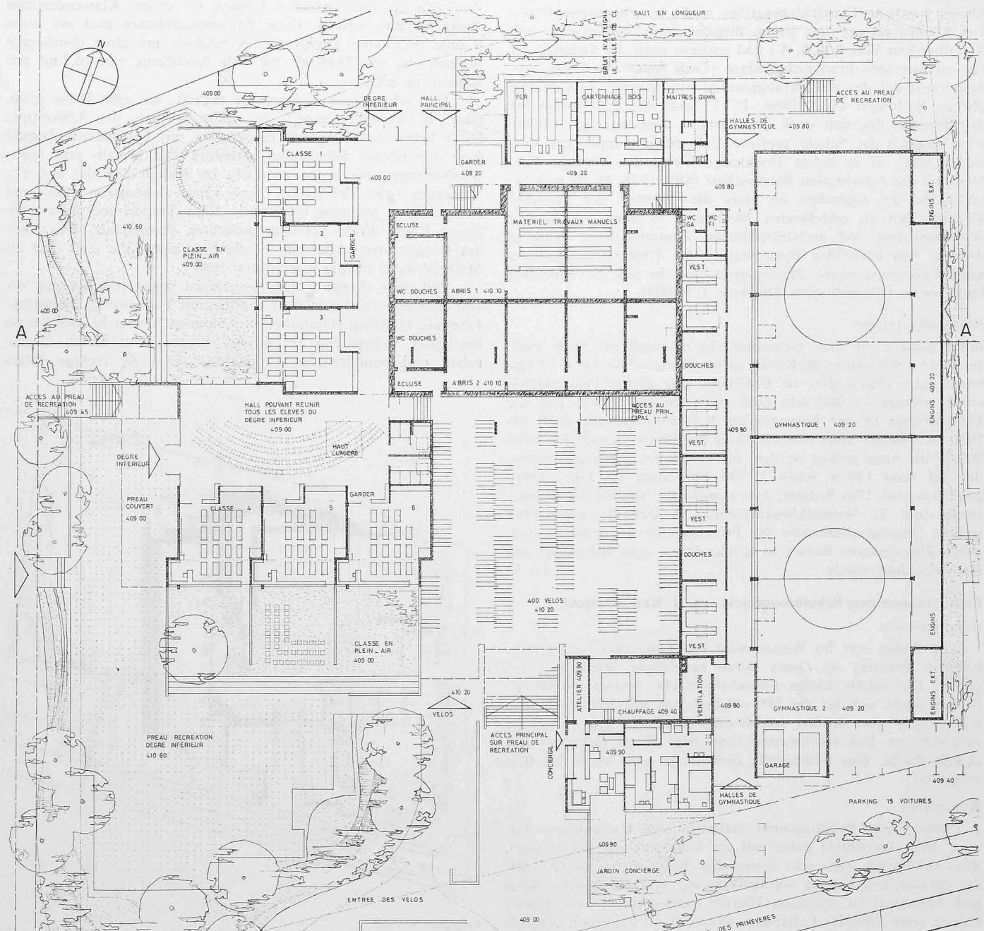
Unteres Eingangsgeschoss 1:500
