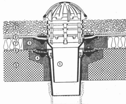
Zweiteiliger Standard-Dachablauf im Kiesschüttung
