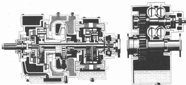
Modernes, vollautomatisches Voith-Differentialwandler-Getriebe
