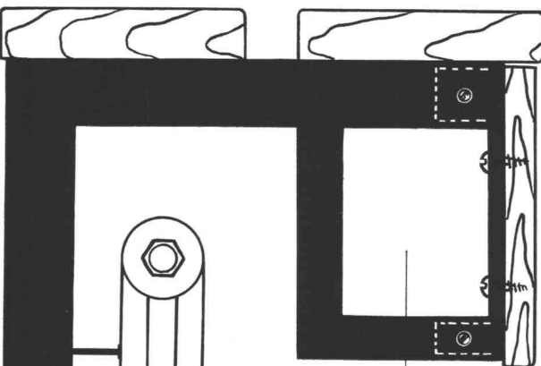
Sitzbank-Konsole mit Radia- torenbefestigung und Kabel- kanalträger. Frontverschalung mit Doppel- Steckmuffe oder Bajonett- verschluss. Wand- oder Bodenverankerung. Richtpreis Fr. 14.— bis 18.— einbrenngrundiert.
