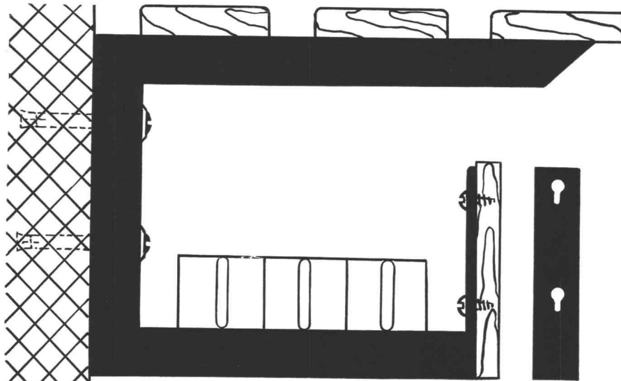
Sitzbank-Konsole mit Konvektorenträger. Frontverschalung auf Bajonettverschluss. Wand- oder Bodenverankerung. Richtpreis Fr. 12.— bis 15.— einbrenngrundiert.
