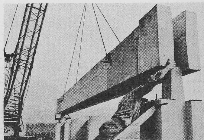
Montage eines Unterzuges
