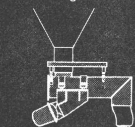
Siloabzug mit Förderrohr
