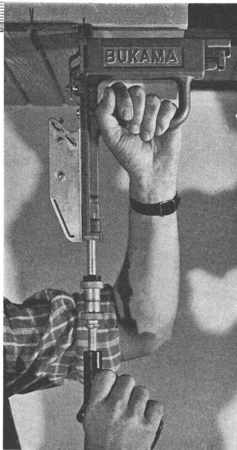
VILIN-Rapid-Aufsatzkopf
