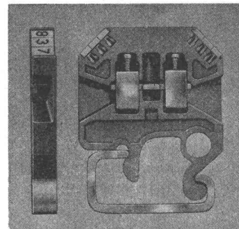
Bild 2. Kleinklemme 2,5 mm 2 , 800 V
