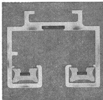
Bild 1. Stromführende Ankerschiene 1 P+N+E, 16 A, 250 V
