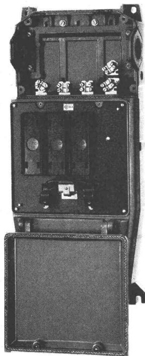
Bild 1. Hausanschlusskasten 3 x 250 A + N
