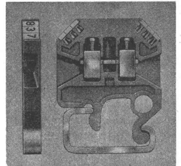
Bild 2. Kleinklemme 2,5 mm 2 , 800 V
