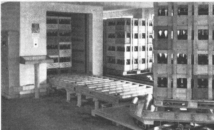
Bild 1. Palettenaufzug; Aufgabe- oder Abnahmestelle mit Be- oder Entladungsmöglichkeit
