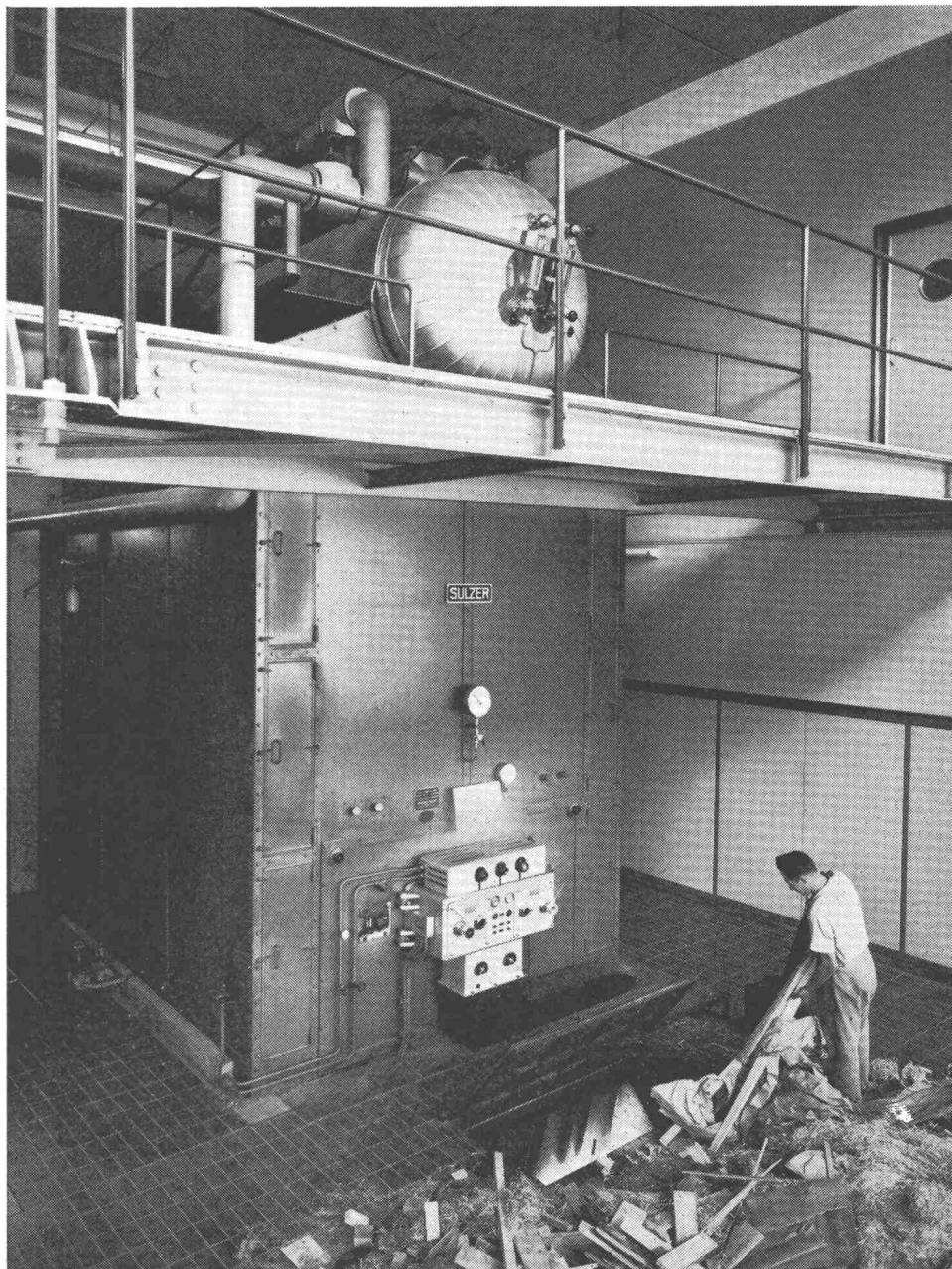
Ölgefeuerter Strahlungskessel Typ C mit einer Vorfeuerung zum Verbrennen von Abfällen. In dieser Anlage einer Maschinenfabrik sind noch zwei weitere Strahlungskessel Typ C aufgestellt. Alle drei Kessel sind für eine höchste Dauerleistung von je 5 t/h und einen Betriebsdruck von 13 atü ausgelegt.
