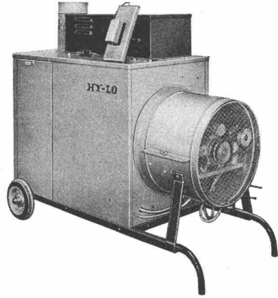
Fahrbarer Luftheritzer Typ K
