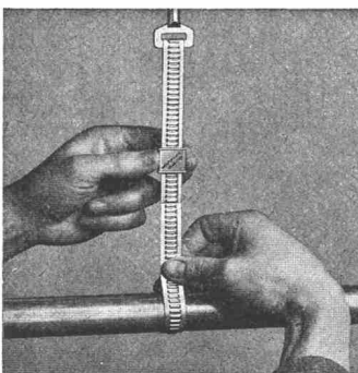
Bild 3. Höhe genau einregulieren und Zahnband eingerastet zusammenrücken.
