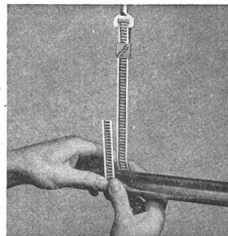
Bild 2. Langes Bandteil sauber um das Rohr biegen, so dass dasselbe ganz umschlossen ist.
