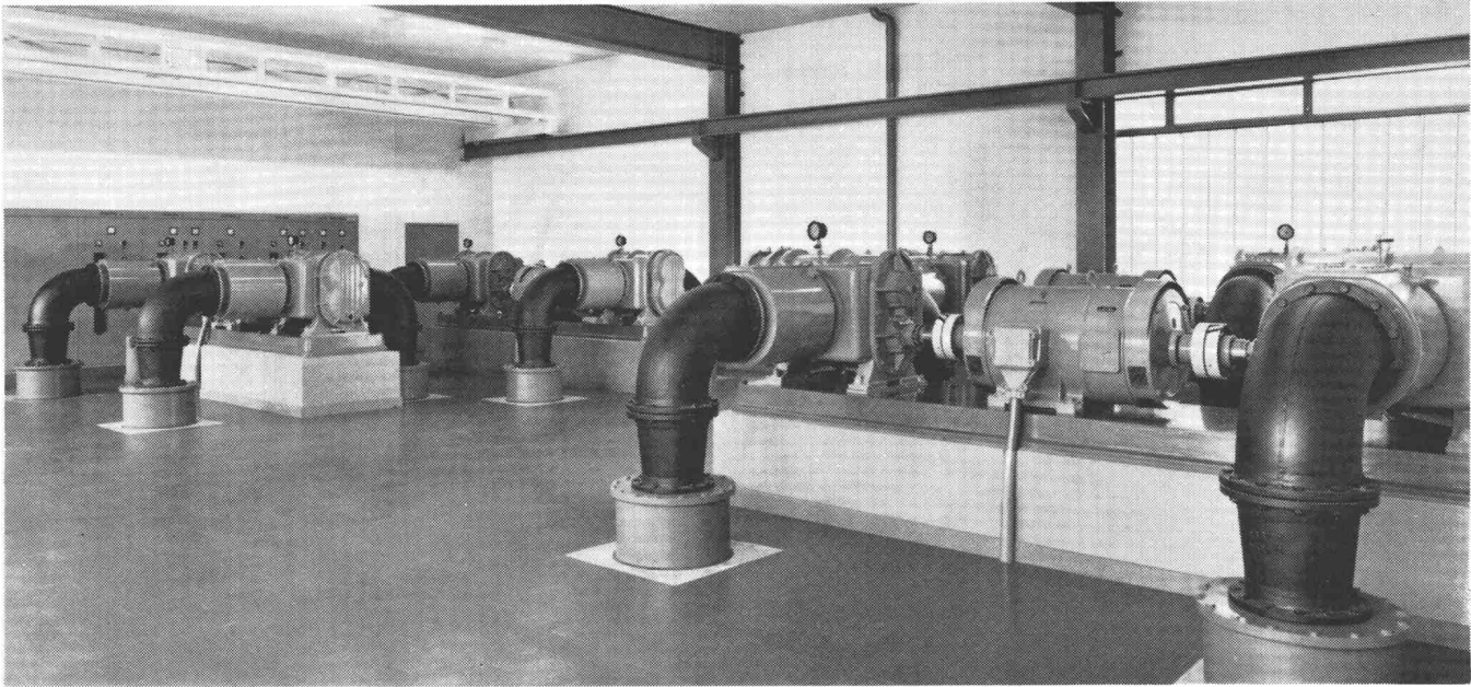
Gebälusanlage, bestehend aus vier Doppelgruppen R 400-400 mit einer totalen Fördermenge von 60 000 m 3 /h, für den Betrieb der Belebtschlammbecken der Kläranlage Hard in Winterthur
