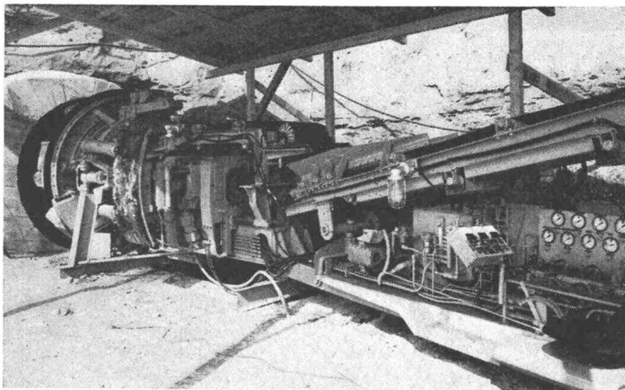
Tunnelvortriebsmaschine Robbins für das Bohren von Stollen in mittelhartem Sedimentgestein.
