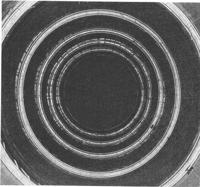
Innenauskleidung eines 100 000 l Stahltanks (Atomkraftwerk Lucens) Revêtement intérieur d'une citerne en acier de 100 000 l (Centrale Atomique Lucens)
