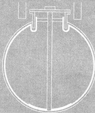
Innenauskleidung eines 100 000 l Stahltanks (Atomkraftwerk Lucens) Revêtement intérieur d'une citerne en acier de 100 000 l (Centrale Atomique Lucens)
