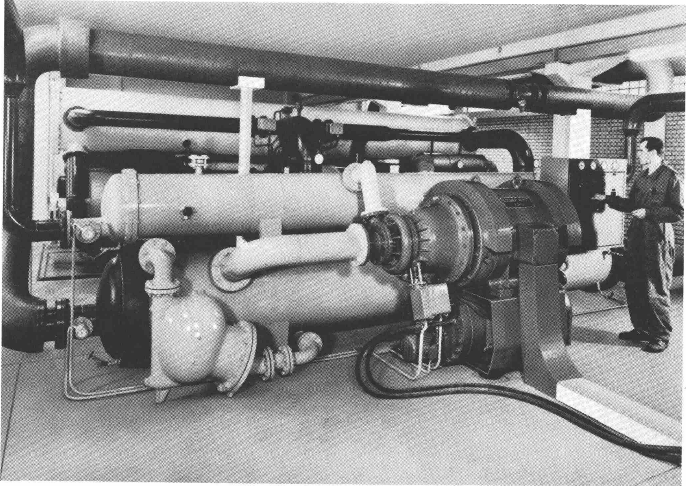
Uniturbo®-Kältesatz Typ 216 mit einer Kälteleistung von 750 000 kcal/h für Wasserrückkühlung in der Klimazentrale des Sulzer-Hochhauses in Winterthur.
