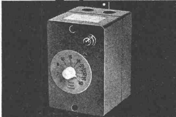
Elektronischer Thermostat zur automatischen Steuerung der Lüfter, gasgeschützt, 220 V~, 3 Amp. 8-40°C Auch für andere Zwecke einsetzbar, da gegen chem. Einflüsse geschützt
