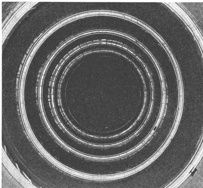
Innenauskleidung eines 100 000 I Stahltankes (Atomkraftwerk Lucens) Revêtement intérieur d'une citerne en acier de 100 000 I (Centrale Atomique Lucens)
