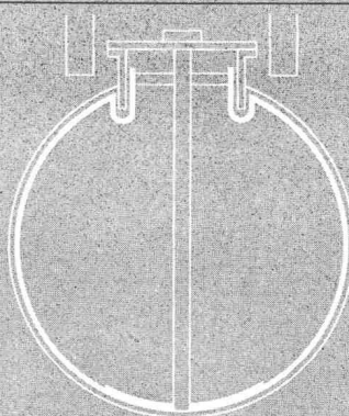
Innenauskleidung eines 100 000 I Stahltankes (Atomkraftwerk Lucens) Revêtement intérieur d'une citerne en acier de 100 000 I (Centrale Atomique Lucens)
