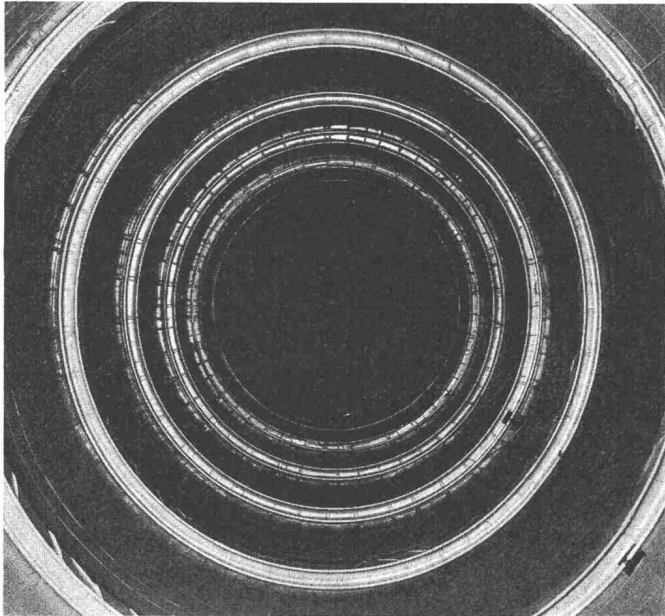
Innenauskleidung eines 100 000 l Stahltankes (Atomkraftwerk Lucens) Revêtement intérieur d'une citerne en acier de 100 000 l (Centrale Atomique Lucens)
