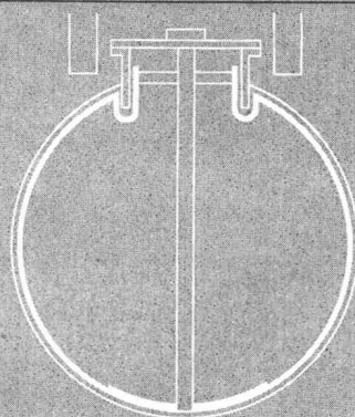
Innenauskleidung eines 100 000 l Stahltankes (Atomkraftwerk Lucens) Revêtement intérieur d'une citerne en acier de 100 000 l (Centrale Atomique Lucens)
