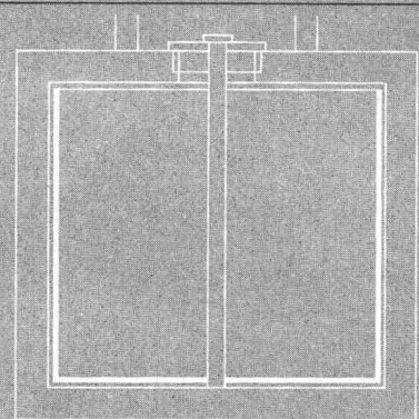
Innenauskleidung eines 250 000 l Betontankes Revêtement intérieur d'une citerne en béton de 250 000 l
