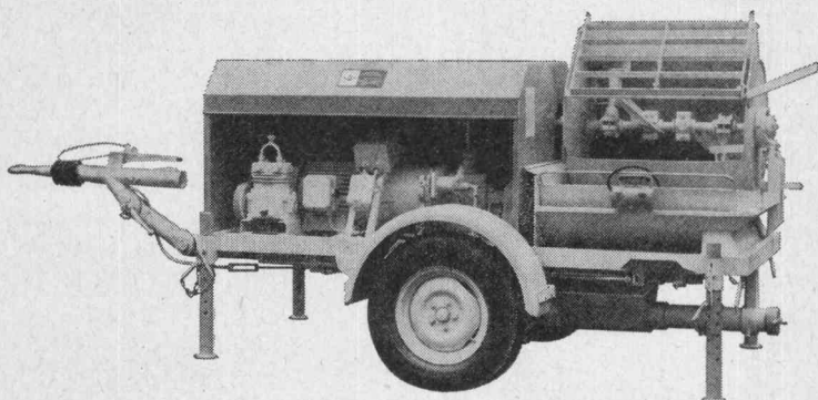
AZAR Typ IE 15 M mit 15-PS-Elektromotor und 200-l-Mischerfüllung. Die Standardmaschine für normal pumpfähigen Mörtel.
