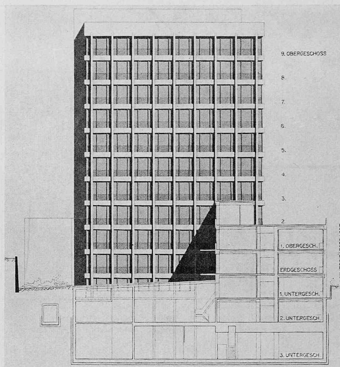
Bild 15. Schnitt A-A 1:600 mit Nordfassade des quergestellten, hochgezogenen Gebäudetракtes. Schnittbezeichnung siehe Bild 13
