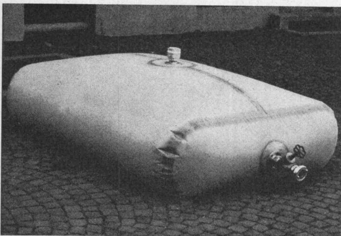
Bild 1. Geschlossener EXCALOR-Fal tank aus Perbunan-beschichtetem Polyestergewebe (Trevira) für Wasser, Öl oder Chemikalien; Fassungsvermögen 1000 l.
