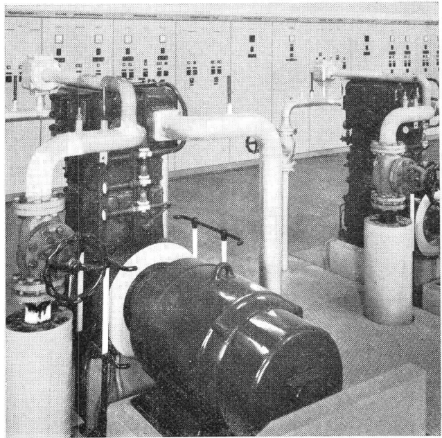
Maschinenraum mit 2 Sulzer-Labyrinthkompressoren für ölfreien Kältemittelkreislauf
