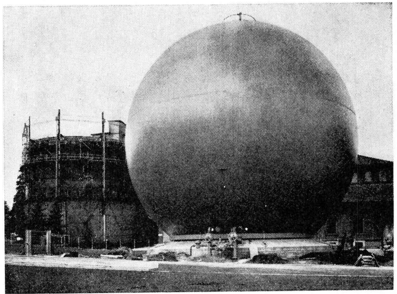
Moderner Hochdruck-Kugelgasbehälter des Gaswerks der Stadt St. Gallen im Riet/Goldach — der erste seiner Art in der Schweiz.
