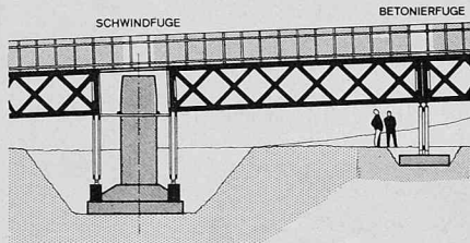
Bild 21. Lehrgerüstkonstruktion
