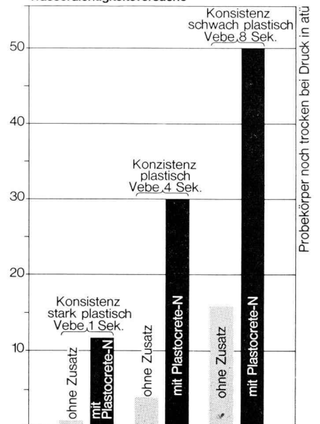
Wasserdichtigkeitsversuche
