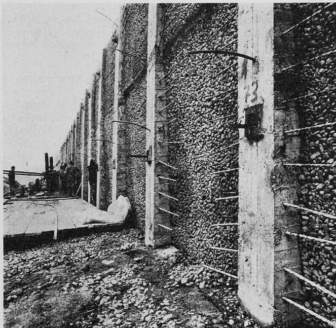
Bild 2. Vorgespannte Riegelstützmauer im Bauzustand. Riegel mit Spannsystem (System VSL) und Sickerbeton
