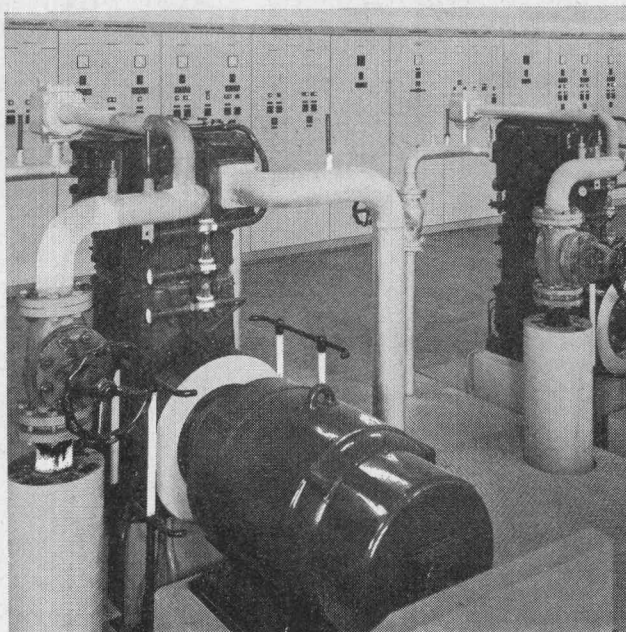
Maschinenraum mit 2 Sulzer-Labyrinthkompressoren für ölfreien Kältemittelkreislauf
