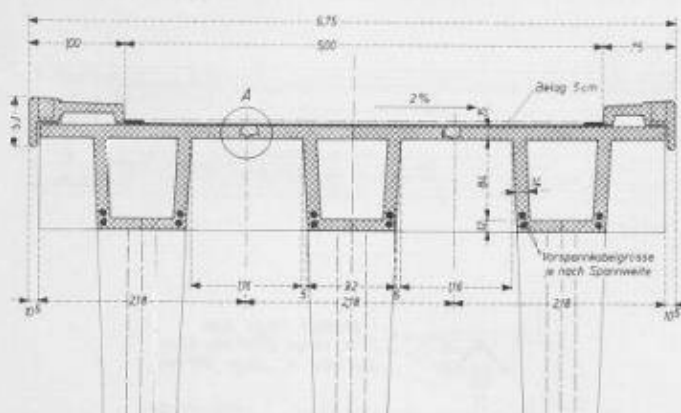
Bild 5. Voll vorfabrizierte Überführung, Querschnitt 1:80. Detail A: Fuge (Asymmetrie wegen Montage)
