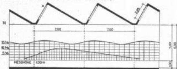
Shedoberlichter mit schrägen Glasflächen Mittelwert 16,6°
