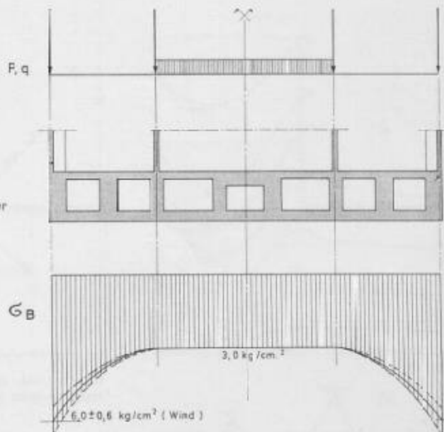
Bild 14b (rechts). Verteilung der Bodenpressungen
