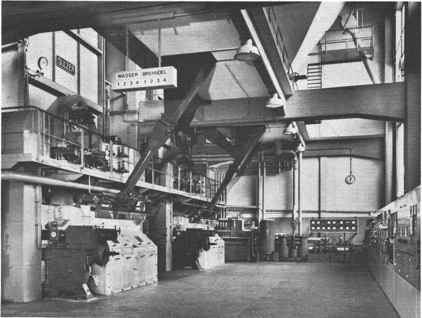
Zwei Strahlungskessel Typ H in einer Maschinenfabrik, ausgerüstet mit Wanderrost- und Sulzer-Ölfeuerung. Dampfmenge je Kessel 20/25 t/h, Druck 34 atü, Temperatur 400 °C.
