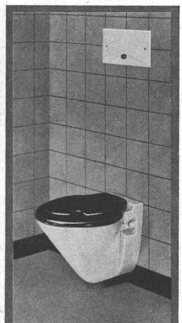
GEBERIT-PVC-Spülkasten für Wandebau Nr. 15.000, mit Anschlussgarnitur Nr. 49.300 für an der Wand befestigtes Klosett
