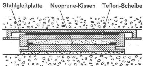
Stahlleitplatte Neoprene-Kissen Teflon-Scheibe
