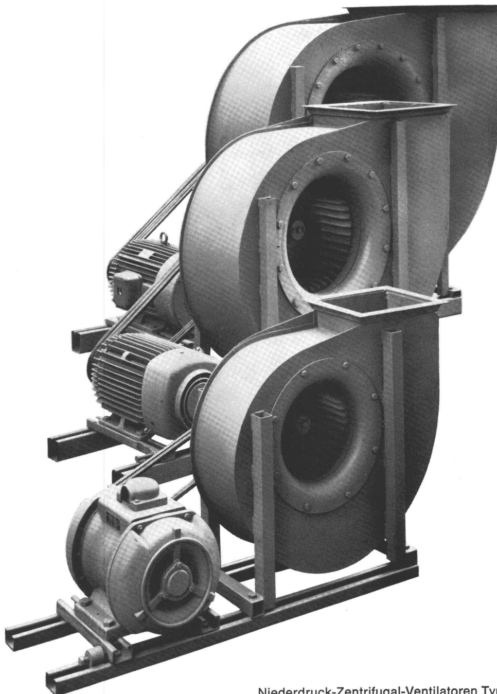
Niederdruck-Zentrifugal-Ventilatoren Typ NVSL
