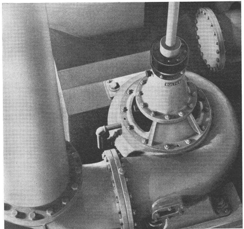
Sulzer-Bohrlochpumpen im Grundwasserpumpwerk Hard II der Wasserversorgung Lenzburg. Jede Einheit fördert 150 l/s auf 132 m.
