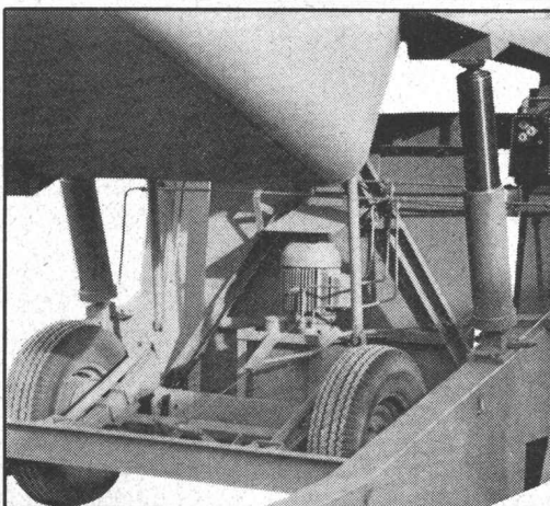
Mech. Absenkvorrichtung
