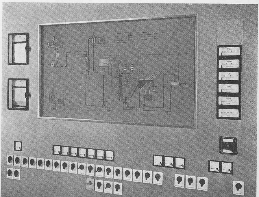
Bild 6. Schalt- und Steuerwarte für eine Escher Wyss-Halbzellstoff-Anlage mit Leuchtschaubild
