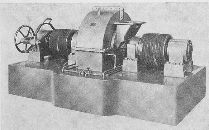
Bild 2. Escher Wyss-Doppelscheiben-Refiner zur Defibrrierung (bzw. zum mechanischen Aufschluss) von Halbzellstoff. Die beiden unter dem Gehäusedeckel angeordneten und mit Mahlsegmenten versehenen Scheiben arbeiten gegenläufig. Stoffeintritt über Zuführtrichter rechts am Gehäusedeckel. Einstellung des Scheibenabstandes über Handrad und Spindel (links).
