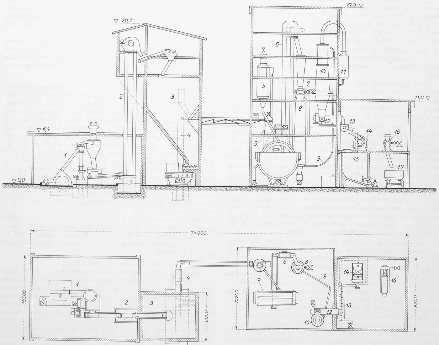
Bild 10. Aufstellungsplan der Anlage nach Bild 9.
