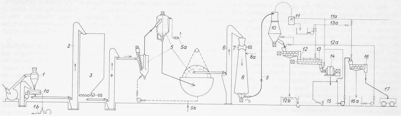
Bild 9. Fließschema einer Halbzellstofffabrik mit kontinuierlicher Escher Wyss-Anlage.
