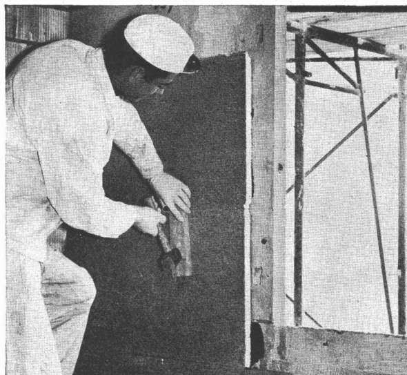
SCHICHTEX 35/III als Innenisolation auf Betonelement aufgeklebt
