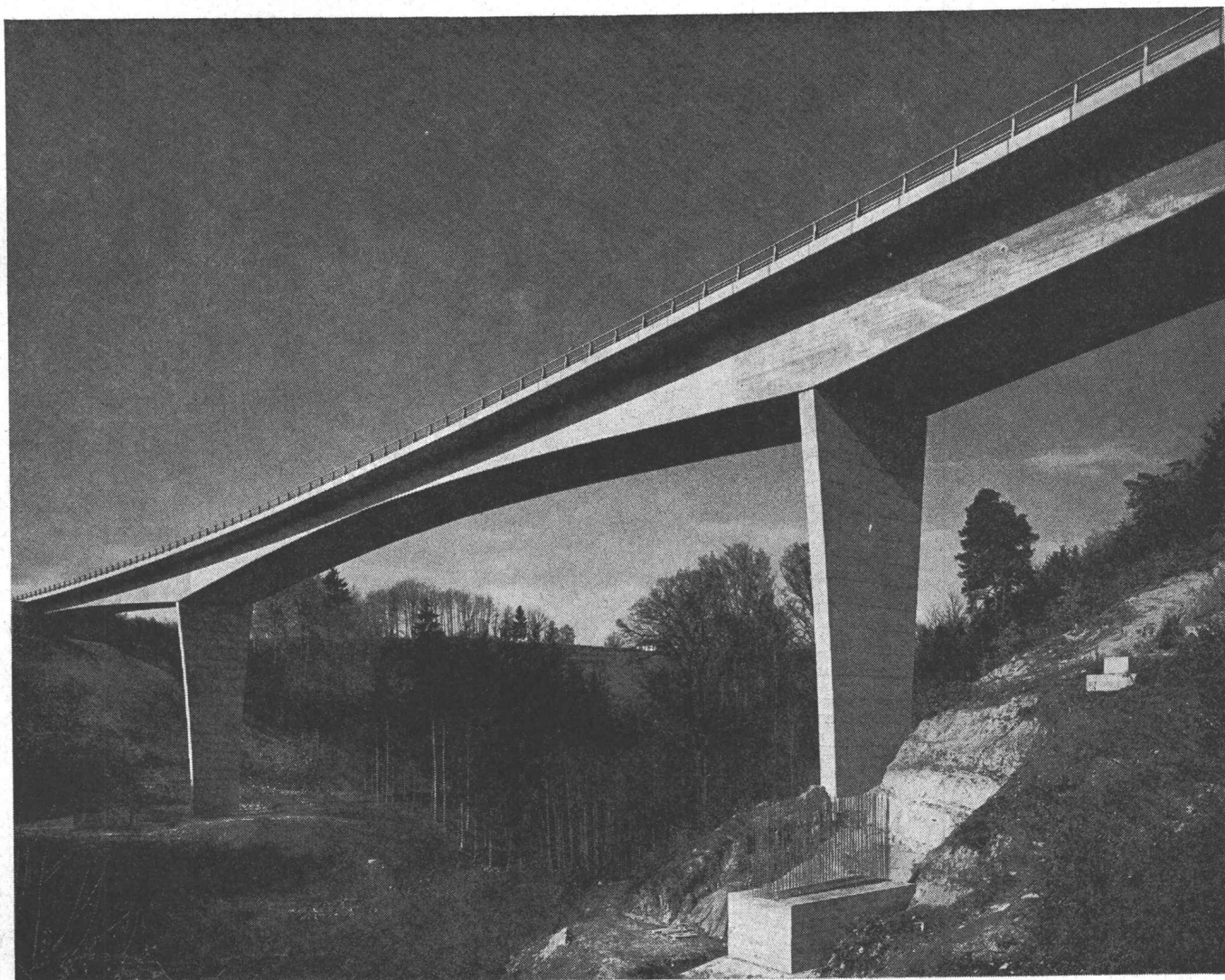
Umgehungsautobahn bei Lausanne: Brücke über die Sorge. Das Bauwerk enthält 11339 m Kabel mit 12 Drähten von 8 mm Durchmesser und 500 Ankerköpfe.
