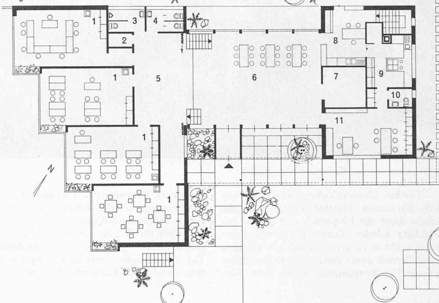
Untergeschoss 1:500
