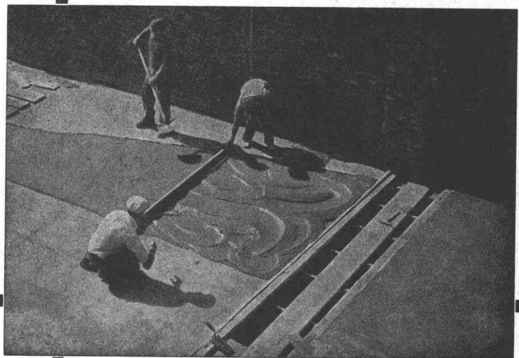
Flachdach im Gefälle, begehbar.
