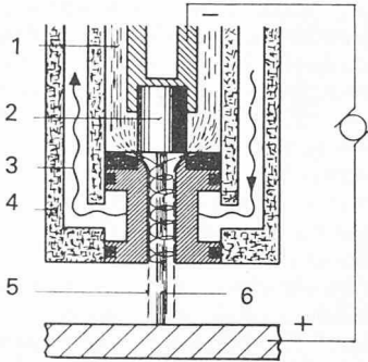
Bild 1. Plasmabrenner mit offenem Lichtbogen (übertragener Lichtbogen)
