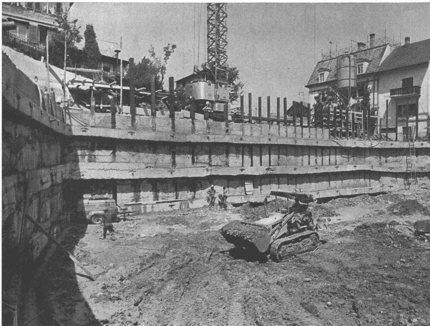
Spriessungsfreie Baugrube
