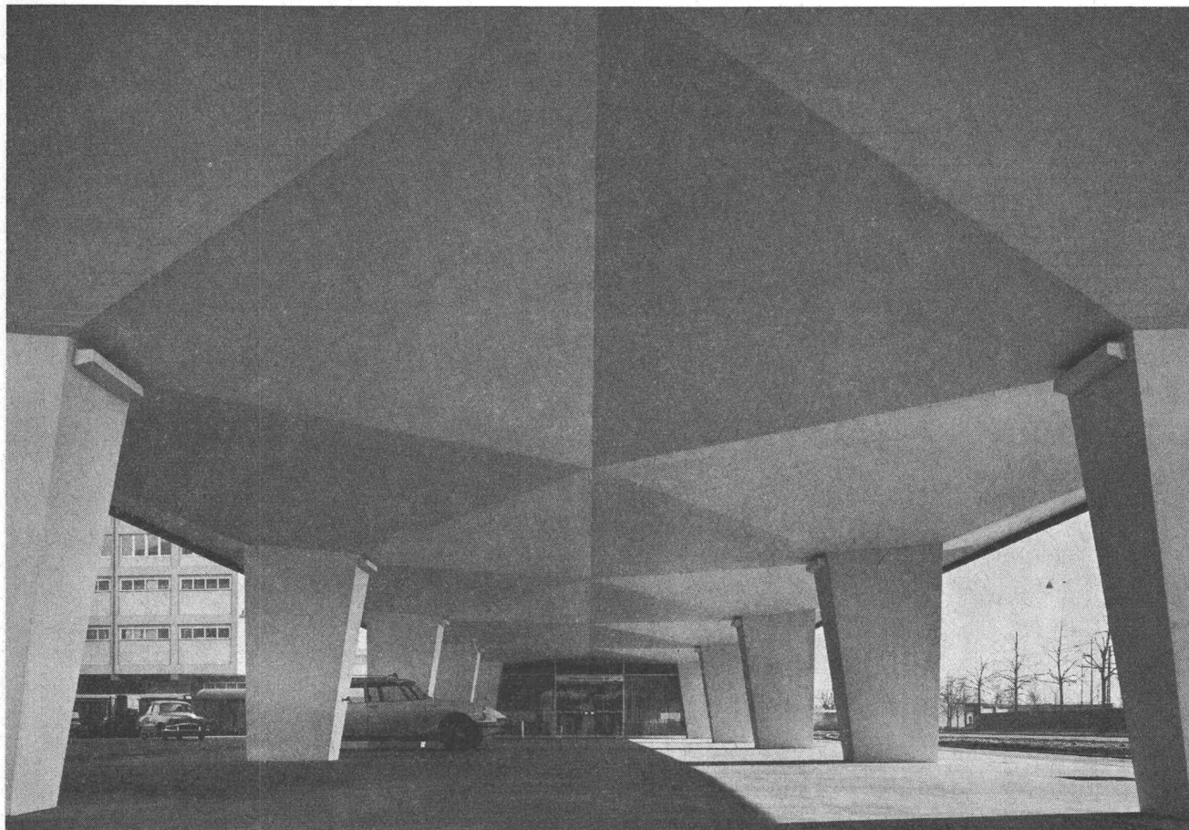
Bau DURAND & HUGUENIN AG, BASEL Massive Pilzdecke, je 450 m 3 Beton ohne Arbeitsfugen eingebracht
