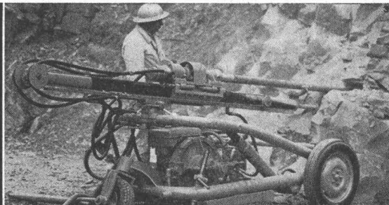
Grosslochbohrwagen mit hydraulischem Antrieb für Lochhämmer
