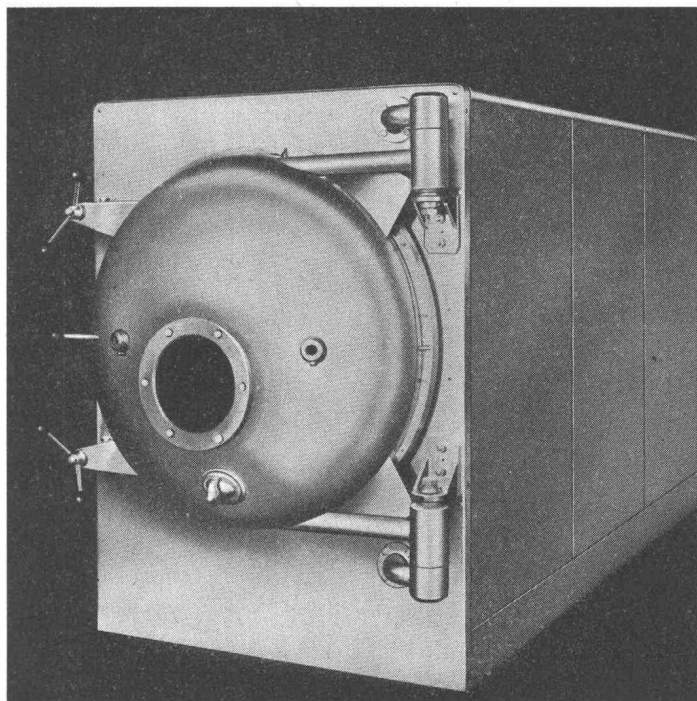
Ygnis-Rayol-Kessel
