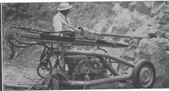
Grosslochbohrwagen mit hydraulischem Antrieb für Lochhämmer
