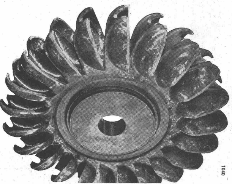
Eines der fünf an die Ateliers des Charnillies S.A., Genf, gelieferten Peltonräder für das Kraftwerk Koyana (Indien) Werkstoff: Chromnickelstahl (13%) Gewicht: 10,5 t Leistung je Turbine: 105000 PS
